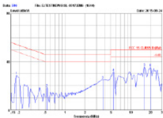
FCC15 CLASS B AV 100V/60Hz 100% LOAD MARGIN: >14 dB
