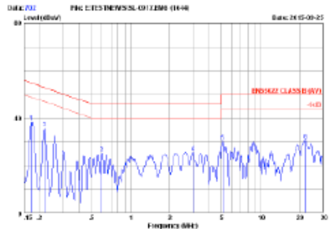
CISPR22 CLASS B AV 230V/50Hz 100% LOAD MARGIN: >16 dB
