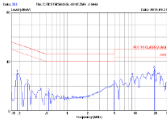
FCC15 CLASS B AV 100V/60Hz 100% LOAD MARGIN: >16 dB
