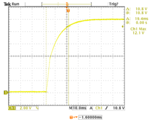
12V Rise Time
