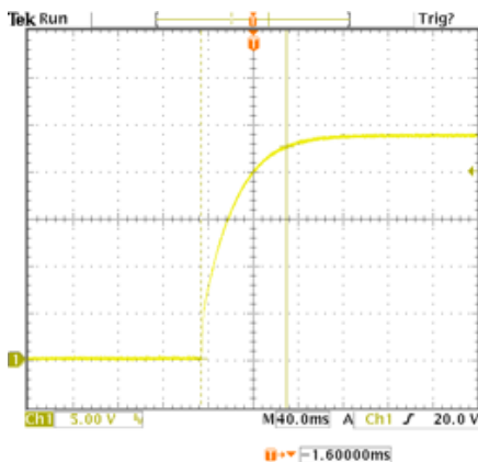
24V Rise Time
